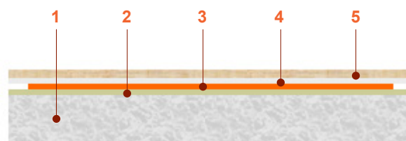
Corte transversal del suelo - calefacción directa
